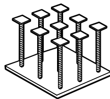
Закладные детали
