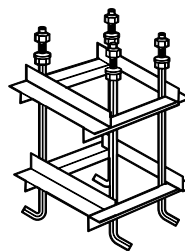
Анкерные блоки
